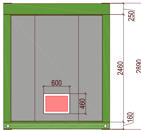
PROSPETTO "B"
