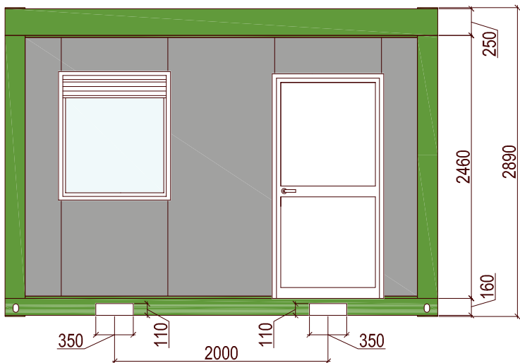
PROSPETTO "A"
